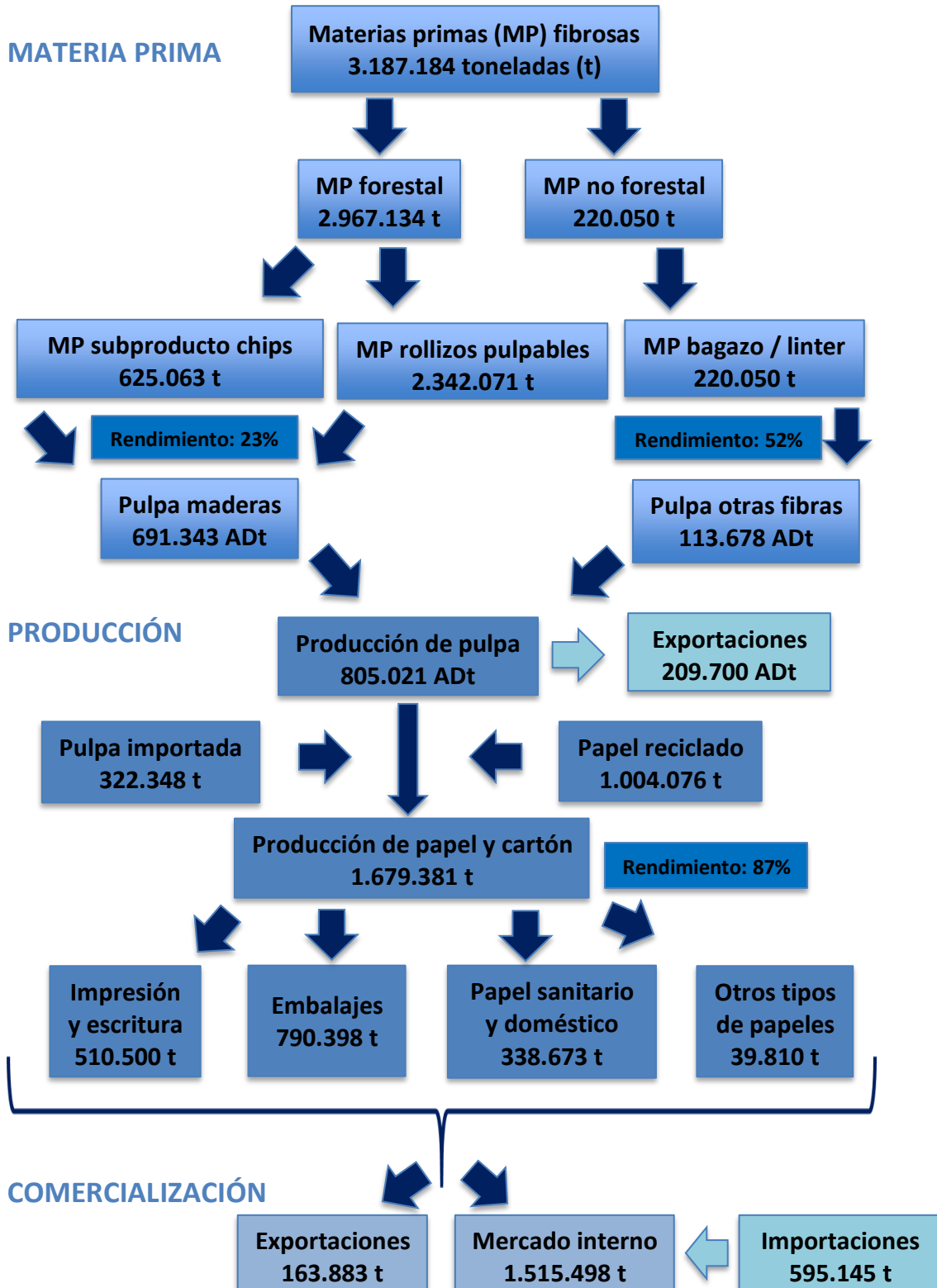
Figura 1: Flujograma de la industria de la celulosa y el papel
